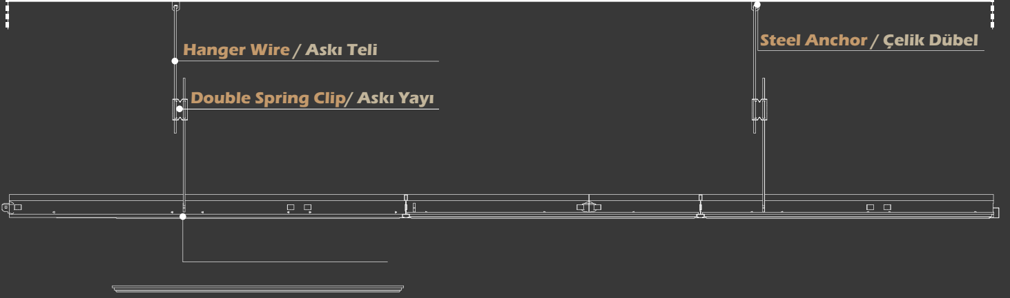
Front / Ön Görünüş
